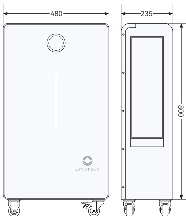
Kích thước Pin lưu trữ LVTOPSUN LVTS-512314-G4
