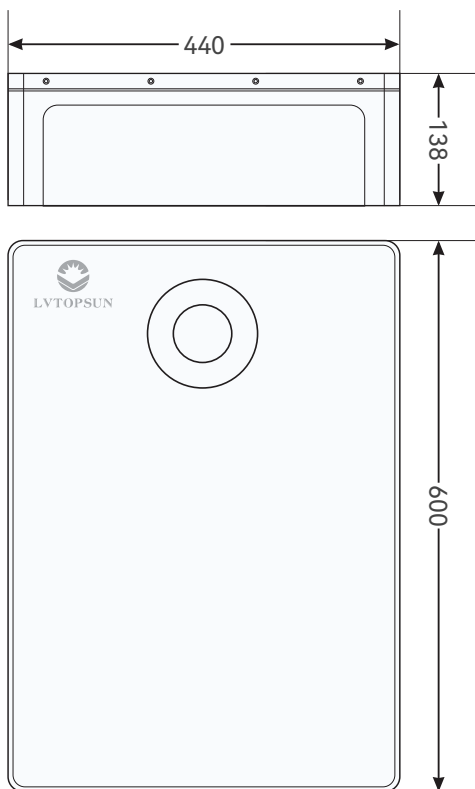
Kích thước Pin lưu trữ LVTOPSUN LVTS-512100-G3
